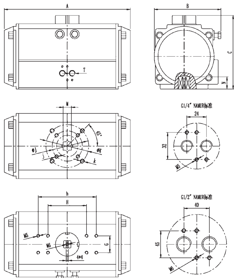
执行机构--尺寸表 ( mm )
