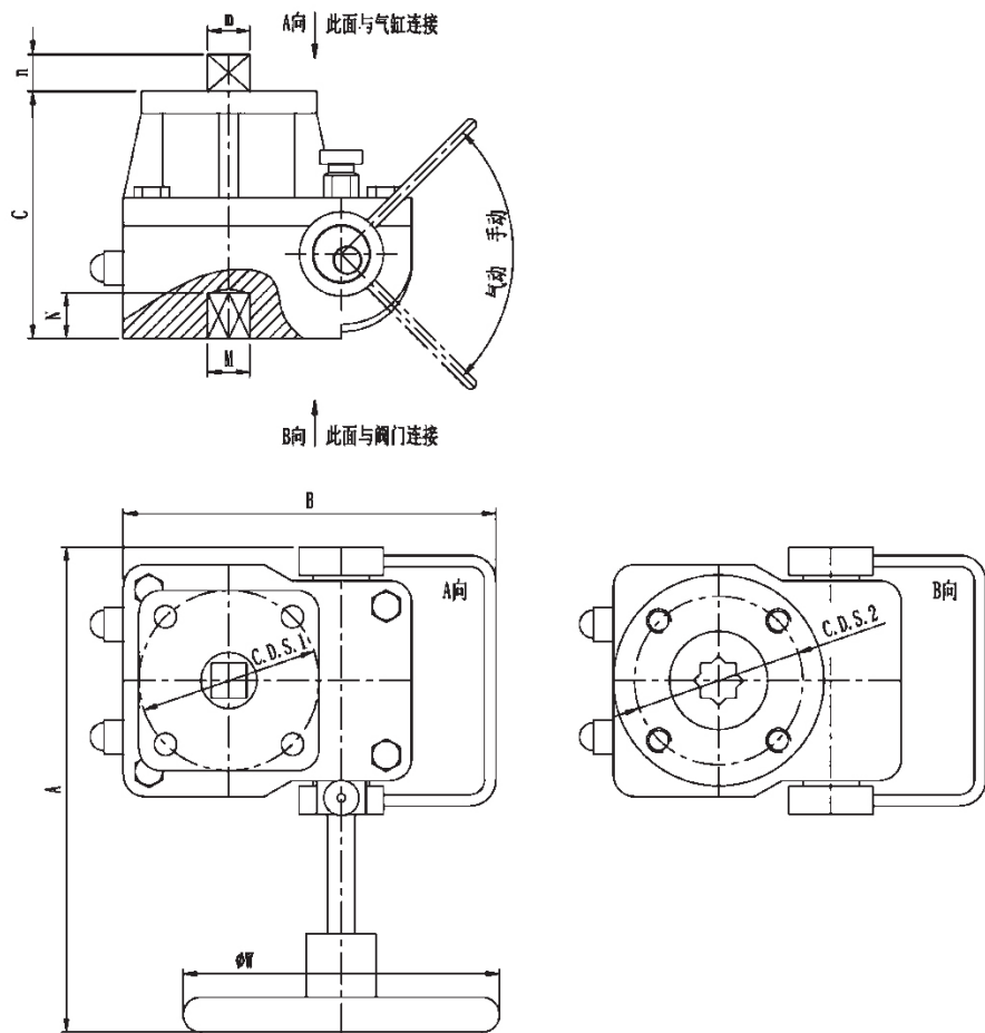
手动机构--尺寸表 ( mm )
